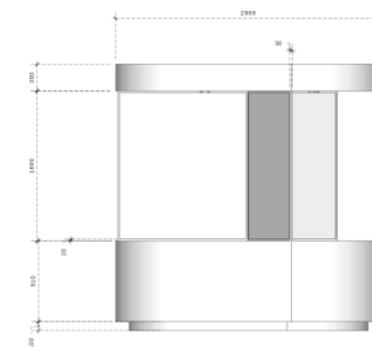
右视图
